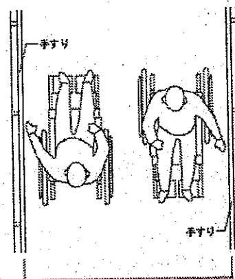
【図3.2】車いす使用者同士がすれ違える寸法 (車いす使用者と杖使用者がすれ違える寸法)
