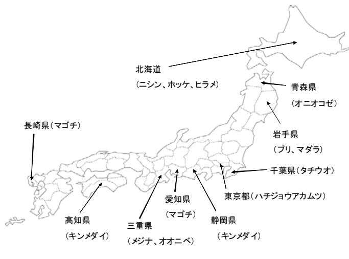
第1図 Anisakis simplex sensu stricto の検出分布
